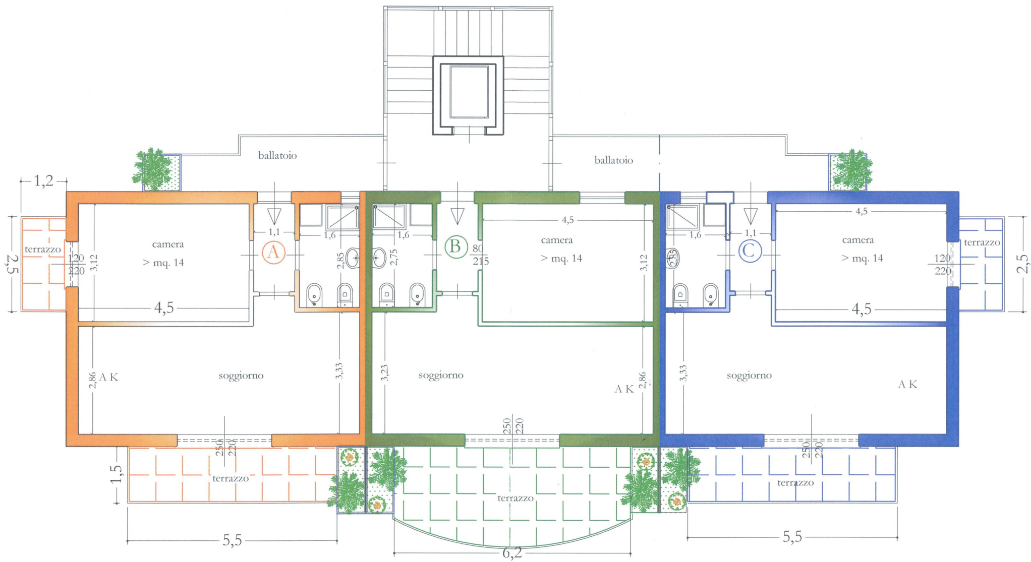
PLANIMETRIA PIANO PRIMO, SECONDO E TERZO
